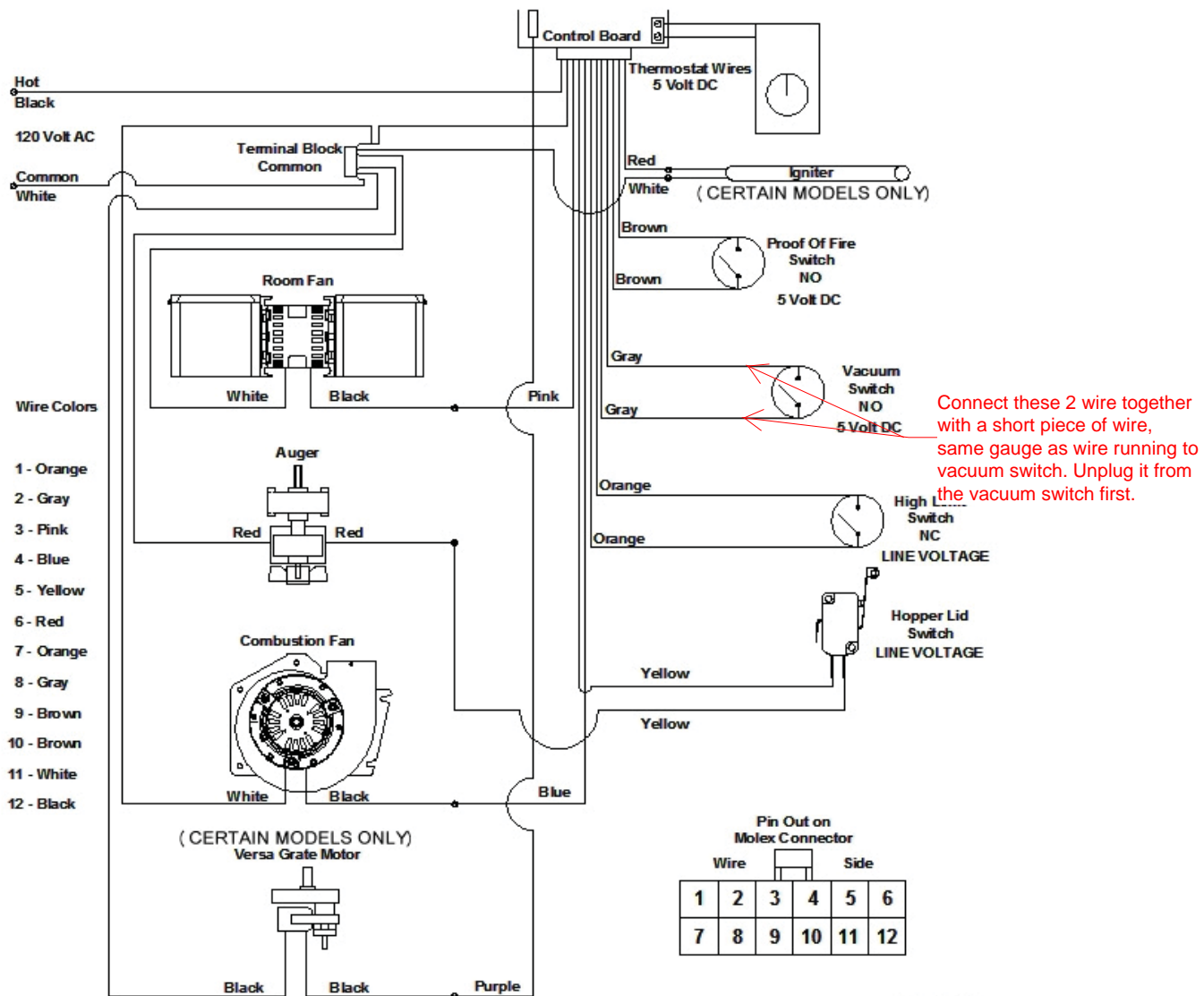
Wiring Schematic
